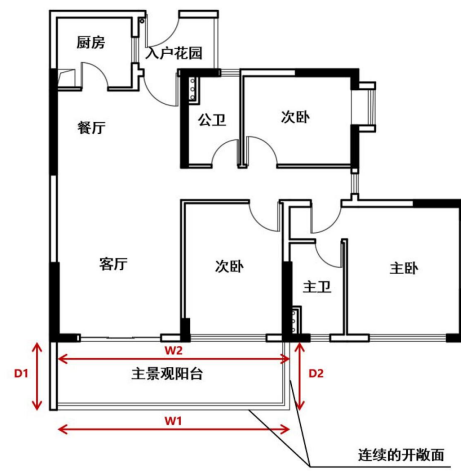
附图 2 主景观阳台及阳台连续开敞率示意图
